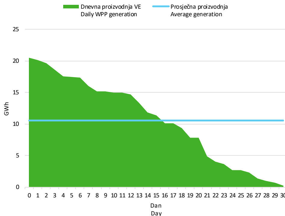
Slika 6 Krivulja trajanja dnevne proizvodnje vjetroelektrana u siječnju 2025. godine
